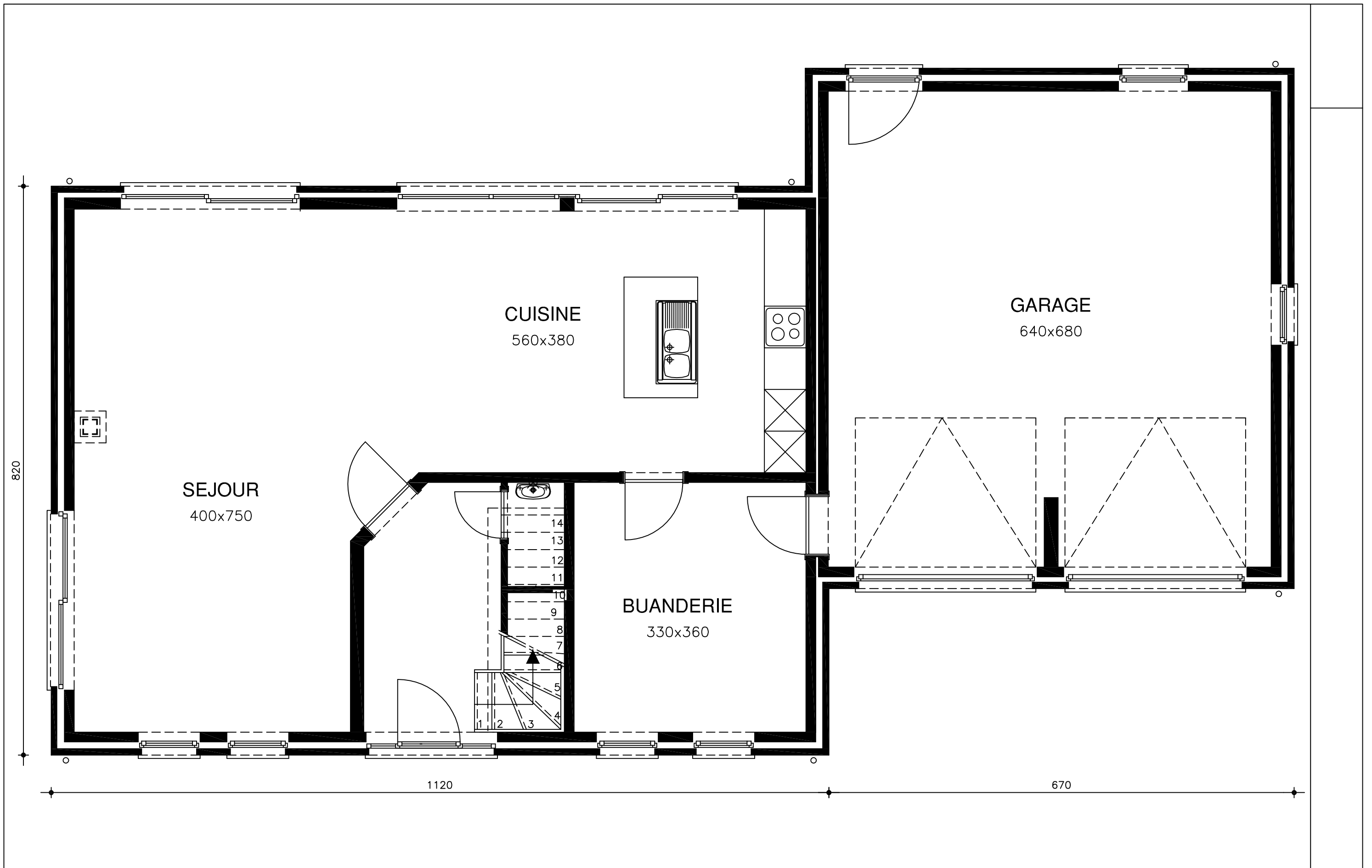
PLAN REZ-DE-CHAUSSEE
