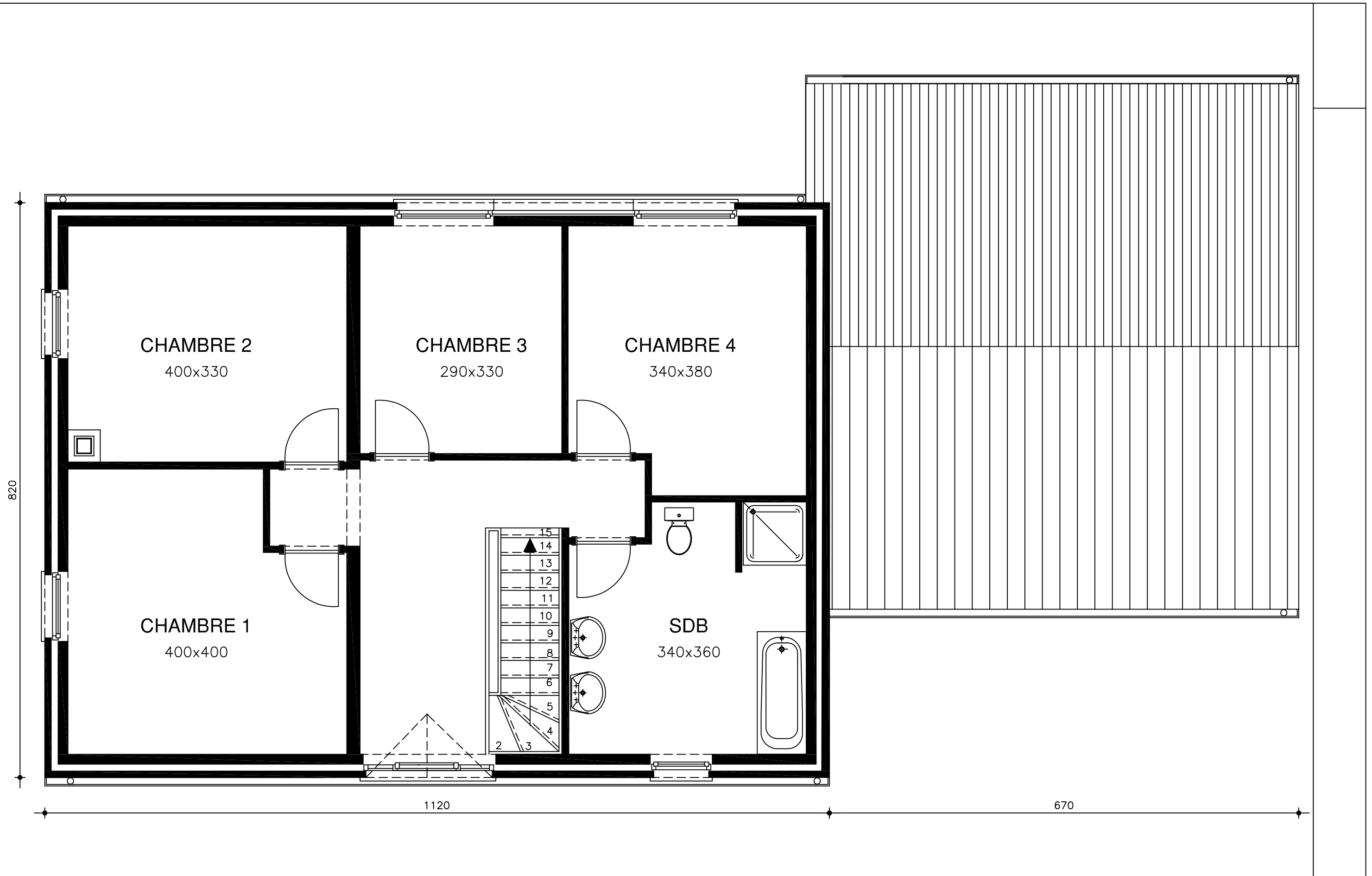
PLAN ETAGE
